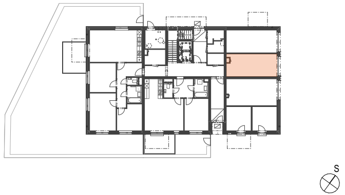
PŮDORYS 1.NP
