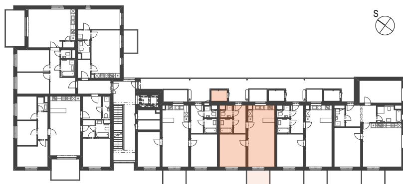
PŮDORYS 3.NP
