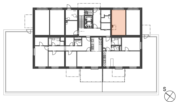
PŮDORYS 2.NP
